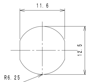
取り付け穴参考寸法
