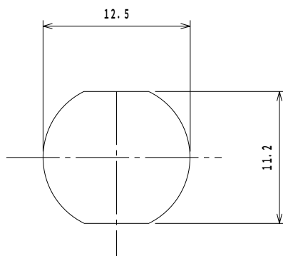
MOUNTING HOLE DIMENSIONS 取付穴参考寸法
