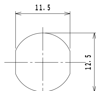
取り付け穴参考寸法
