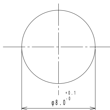
取付穴参考寸法 MOUNTING HOLE DIMENSION
