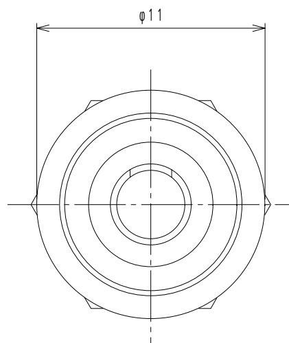
取付穴参考寸法 MOUNTING HOLE DIMENSION
