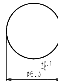
取付穴参考寸法 MOUNTING HOLE DIMENSION
