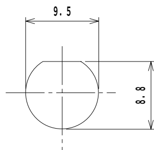
取り付け穴参考寸法 MOUNTING HOLE DIMENSION
