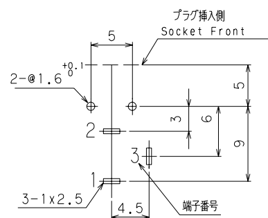
基板穴寸法図 t1.6 mm (半田面より見る BOTTOM VIEW)
