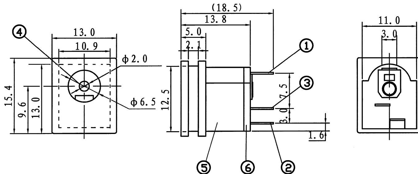
电路结构示意图
