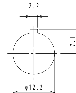
取り付け穴参考寸法
