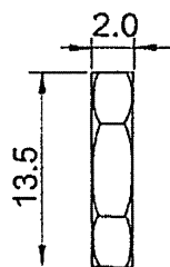
HEX NUT
