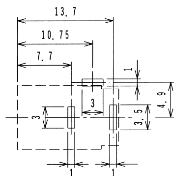
フ°リント基板孔参考図
