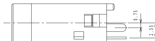
A - A' 断面 A - A' SECT
