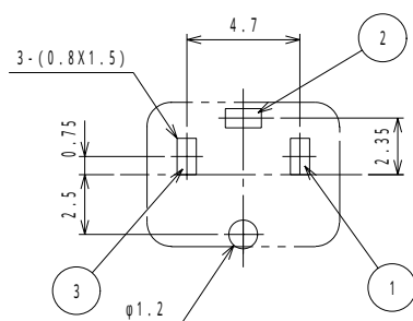
プリント基板参考図 HOLE LAYOUT
