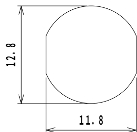
取付穴参考寸法 MOUNTING HOLE DIMENSION
