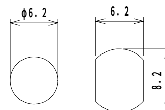
取付穴参考寸法
