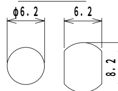
取付穴参考寸法
