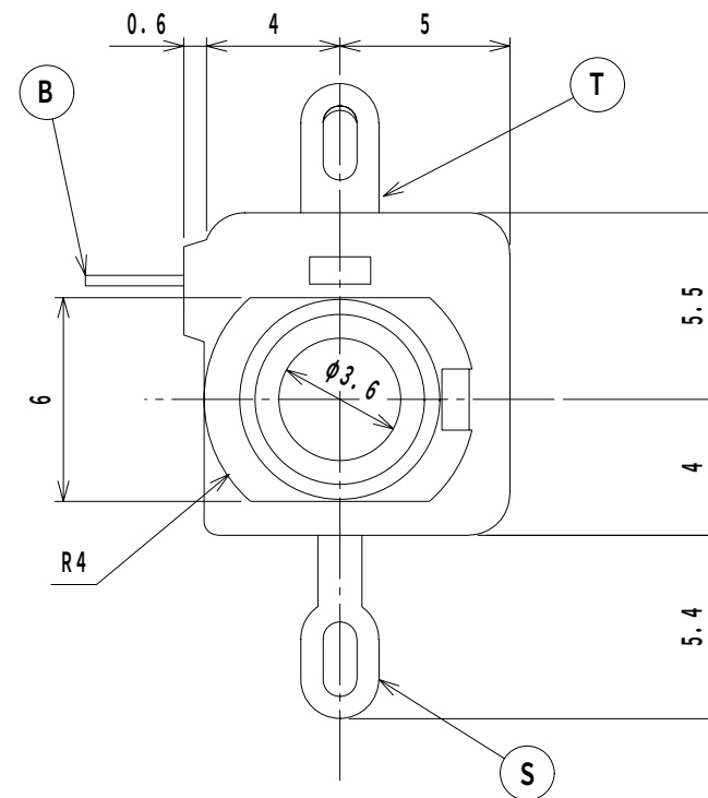
取付穴参考寸法
