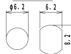
回転止使用時 (板厚 t=0.7 以上)
