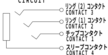
回路図 CIRCUIT
