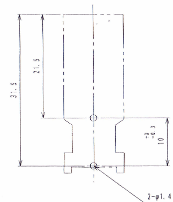
プリント基板参考図
