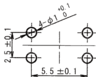
基板取付穴寸法参考図 PC Board hole layout
