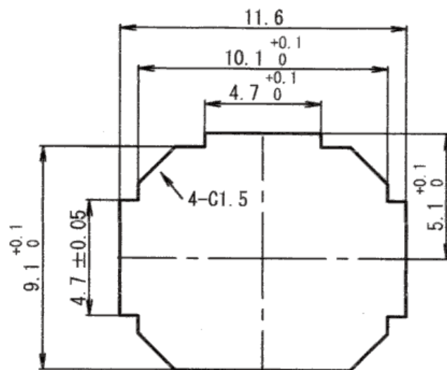
パネル取付穴寸法参考図 Mounting hole dimension
