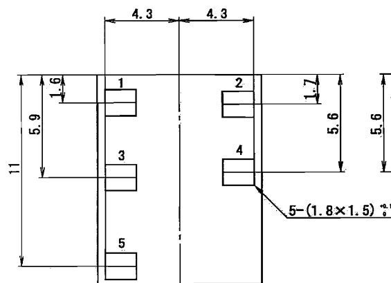
推奨ランド参考図 (公差±0.1mm, 実装面側より見る) Reference drawing of recommendation land (Tolerance ±0.1mm : Seen from mounting side.)
