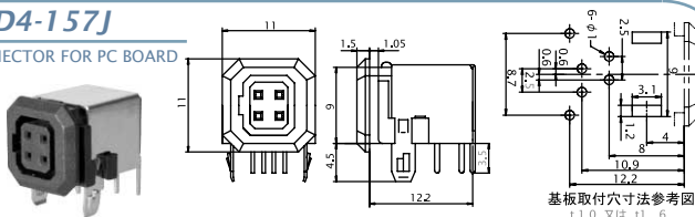
基板取付穴寸法参考図 (t1.0又はt1.6)
